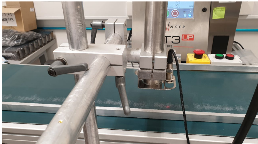
Slika 4: Ročni vijaki za nastavev tiskalne glave
