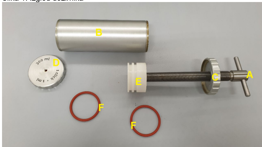
Slika 2: Razstavljen dozirnik
